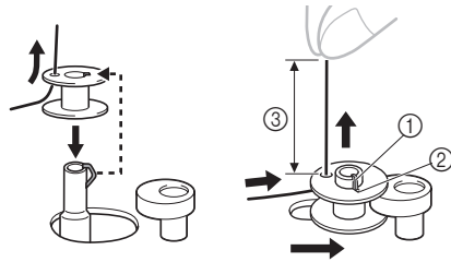
1 Пружина на валу 2 Выемка 3 7–10 см
