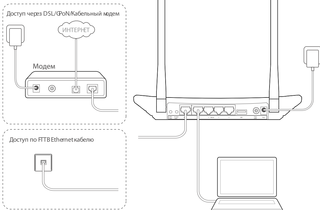
Рис. 2-1 Подключение устройств
