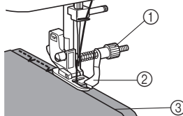
① Винт ② Направляющая ③ Подогнутый край
