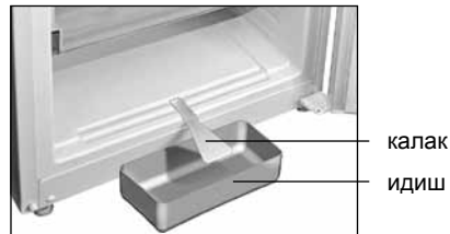
7-сүрөт — ТБ эриген сууну чогултуу
