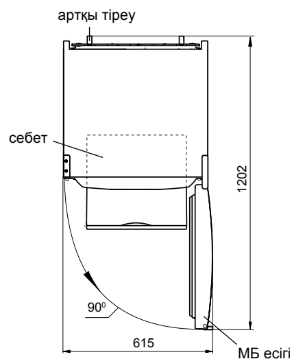
2 сурет — Тоңазытқыш (жоғарыдан көрініс)
