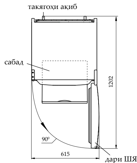
Расми 2 — Яхдон (намуди он аз қисми боло)
