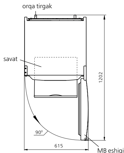
2 rasm – Sovutgich (tepadan ko'rinish)
