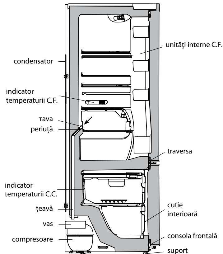
Figura 6 — Schemă de scurgere de apă topită din C.F.
