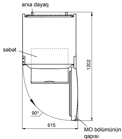
Rəsim 2 — Soyuducu (üstədən görünüşü)
