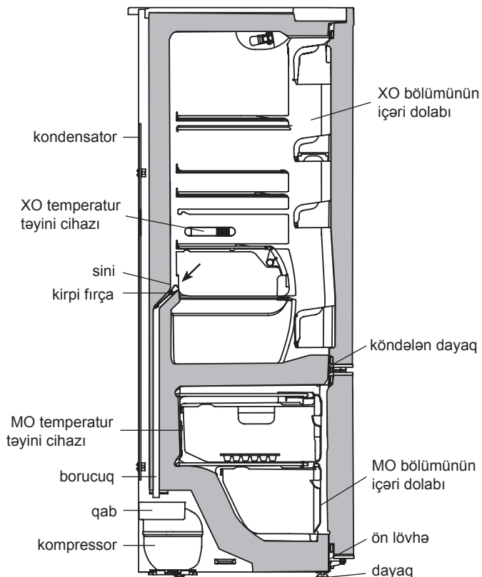
Rəsim 7 — XO bölümünün ərmiş axıntı sularının tökülməsi sxemi
