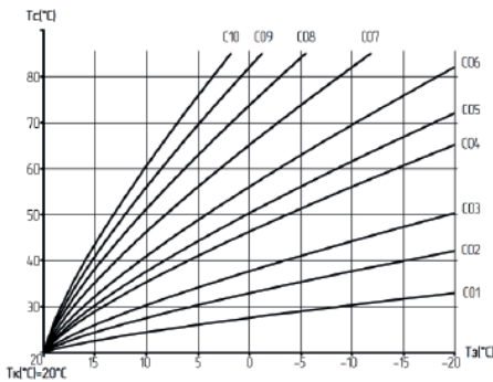
Рисунок 25 Компенсаційні криві
