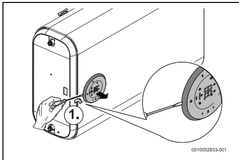
Мал. 12 Виймання дисплея
