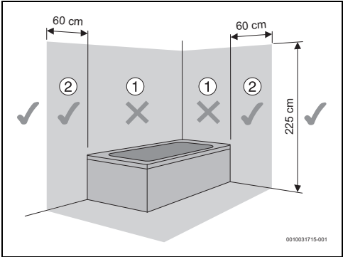
Мал. 7 Захисна зона
