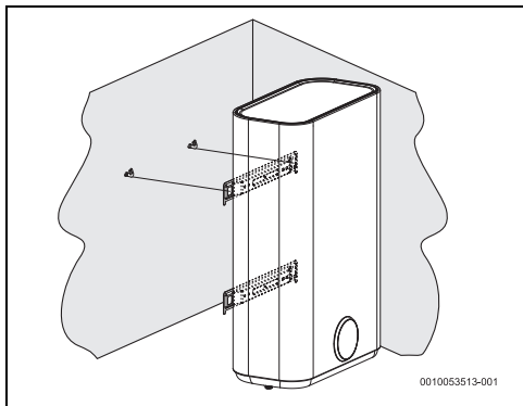
Мал. 9 Вертикальне встановлення (настінний монтаж)
