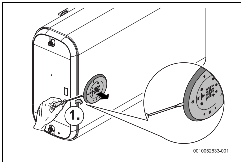
Мал. 11 Виймання дисплея
