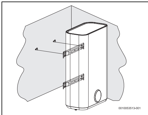
Мал. 8 Вертикальне встановлення (настінний монтаж)
