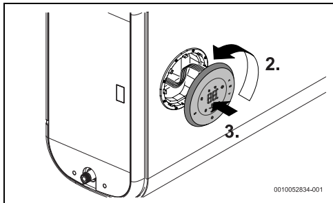
Мал. 12 Повертання і встановлення дисплея
