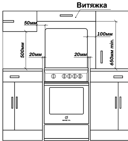
Мал. 1 Установка плити між меблями
