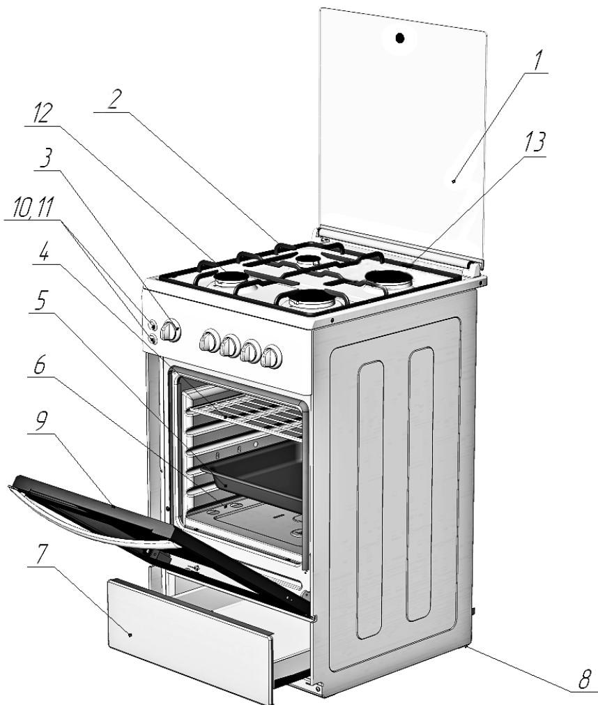
Рис. 7 Устройство плиты
