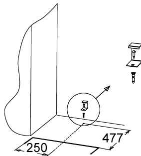
Мал. 2 Розмітка підлоги для установки запобіжного кронштейна
