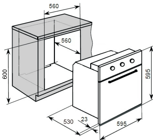
Розміри виробу
