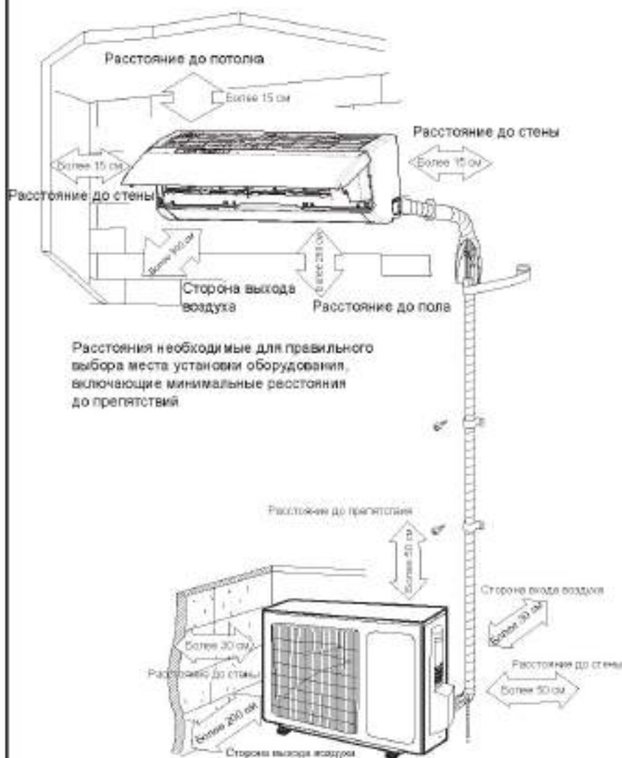
Схема установки
